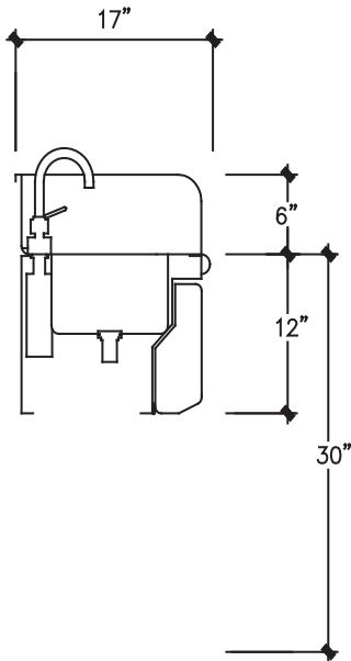
SECTION (WALL MOUNT)
